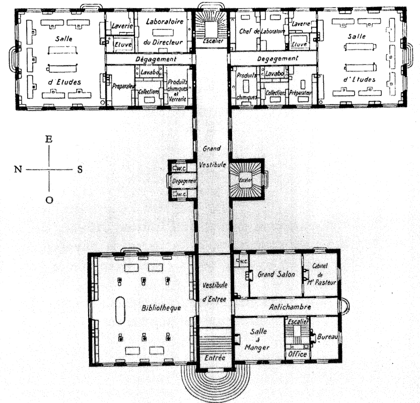
Plan du 1 er étage de l'Institut Pasteur en 1888.
